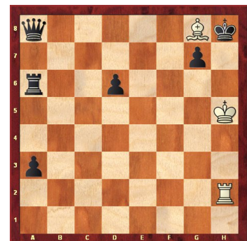
Salkind 1913: Remis
