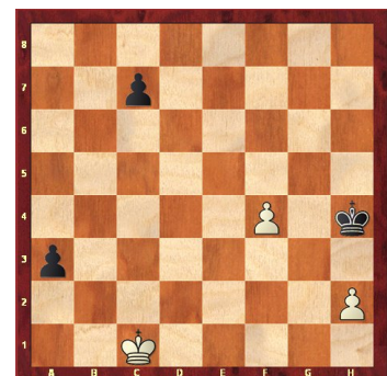
Grigorjew 1937: Gewinn
